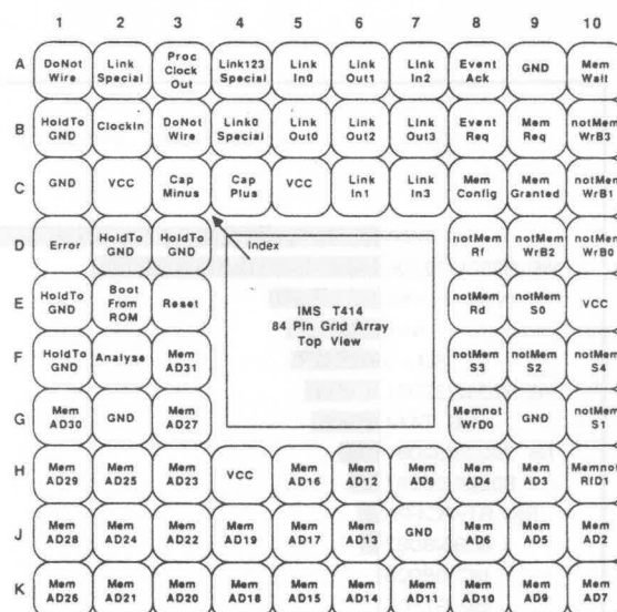
Figuur 1: Pin-layout van de INMOS T414
