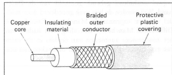
Fig. 3: doorsnede van een coaxkabel
