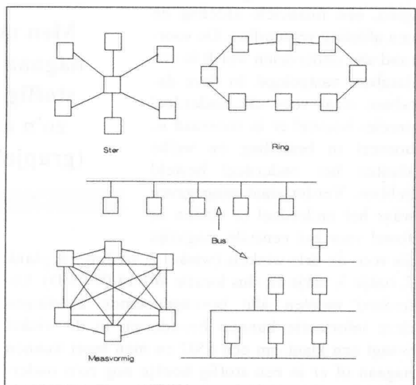
Fig. 1: enkele netwerktopologieën
